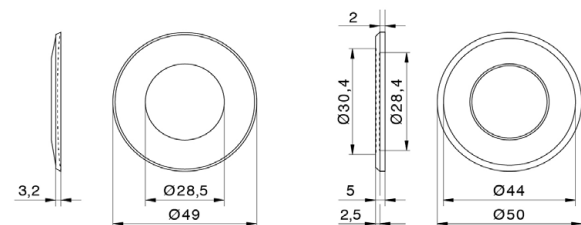
rozeta 50 mm
