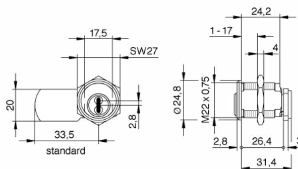
vzor pro montážní otvor
