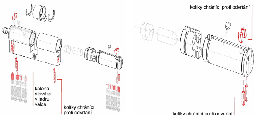
kolíky chránící proti odvrtání
